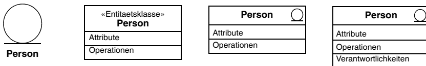
Abb. 24–2 Darstellungsvarianten einer Entitätsklasse
