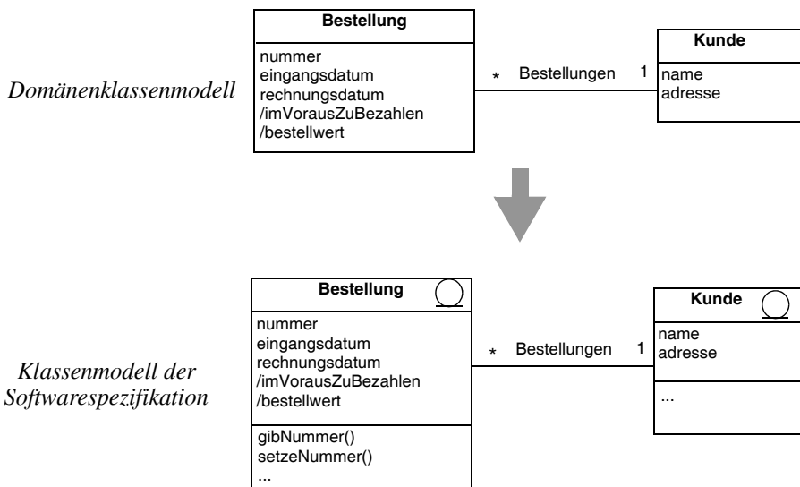
Abb. 24–3 Transformation zweier Domänenklassen in Entitätsklassen im Bestellwesen
