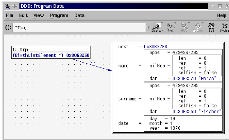
Abbildung 6.6 Mit SHOW ALL können Sie sämtliche Daten einer verschachtelten Struktur expandieren.
