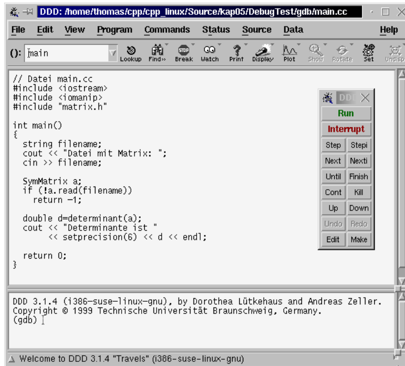
Abbildung 6.1 Die Benutzeroberfläche des DDD bietet einfachen Zugriff auf alle häufig benötigten Funktionen.
