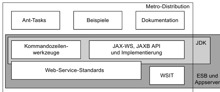
Abb. 4-1 Welcher Bestandteil von Metro ist wo enthalten?
