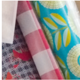
ISO 6400
